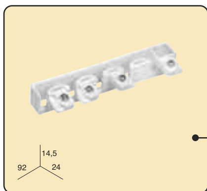
Embout 5 voies
