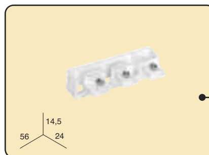
Embout 3 voies
