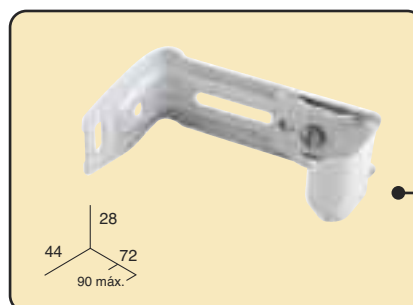
Jeu support central "E" 6-9 cm. (large et étroit)
